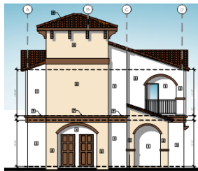
SIDE ELEVATION (BUILDING B1)
