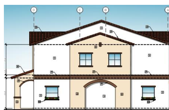
SIDE ELEVATION (BUILDING A)
